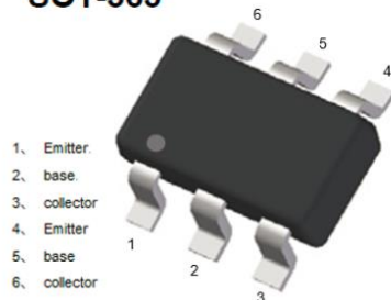
SOT-363
